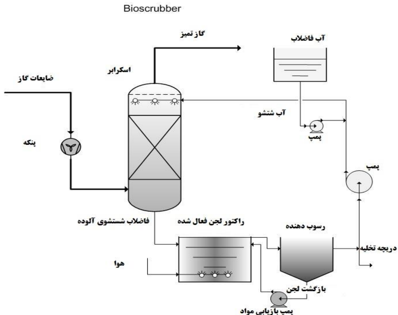
شکل شماره ۱۷. تصفیه هوازی ضایعات گازی با بیواسکرابر
